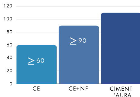
Temps de début de prise sur pâte pure (en minutes)
