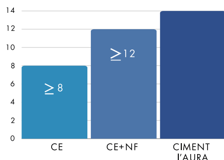
Résistances mesurées sur mortier normalisé (en MPa)
